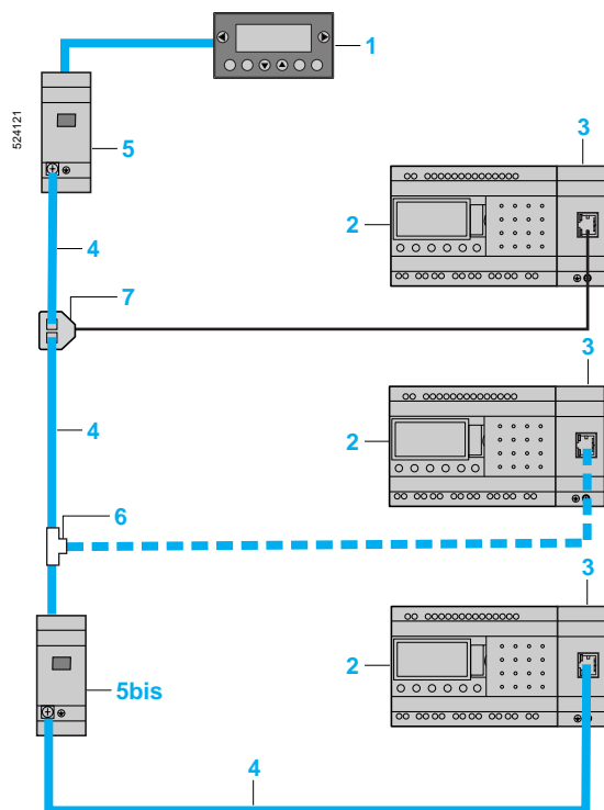
Modbus communication module
